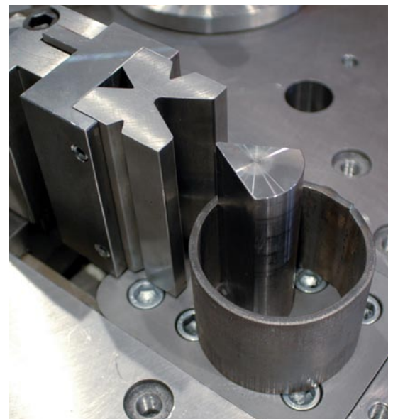
Rundbiegen um Biegedorn
