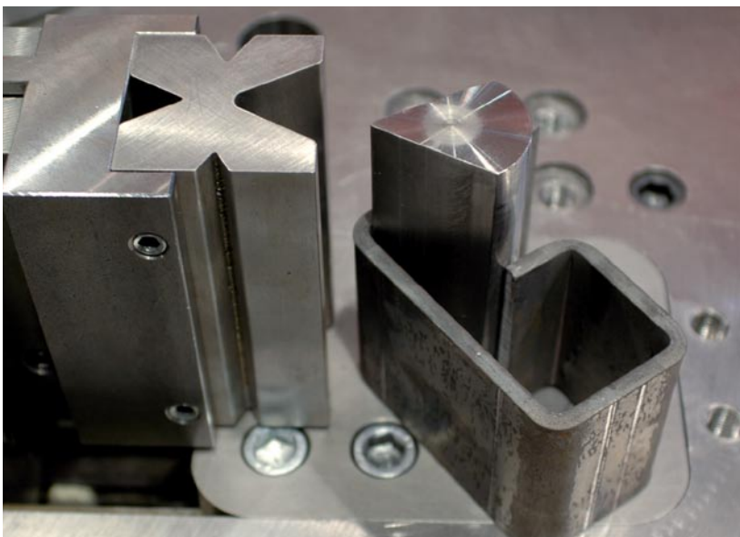
Mindestquerschnitt 50 x 50 mm
