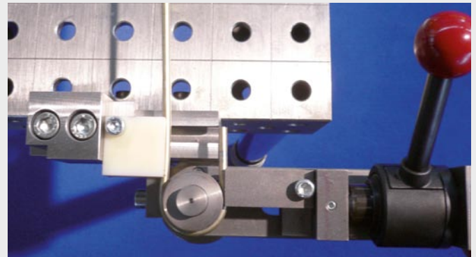
Mindestausführung ohne Messsystem und Verdrehung.
