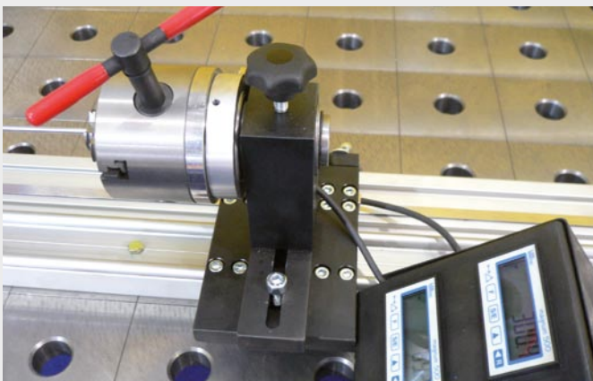
Digitalanzeige für Längenmessung und Verdrehung. Optional: Dornstange mit Rückzug f. dünnwandiges Rohr
