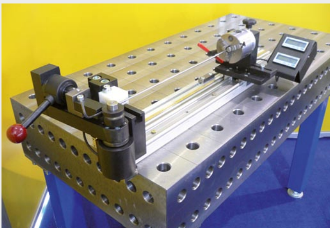
HRB 12-Plus mit 5 mm Draht. Ausstattung mit Messsystem und Verdrehung. Schweißstisch optional.
