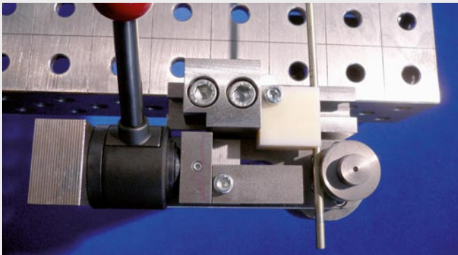
HRB 12 mit 6 mm Rohr. Schweißstisch optional.
