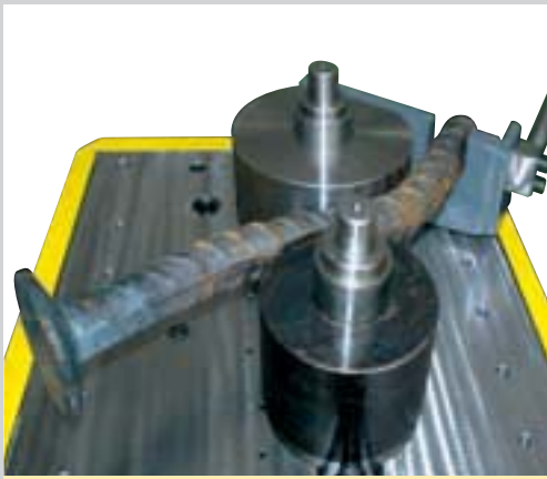
Buigen van staven tot 40 mm
