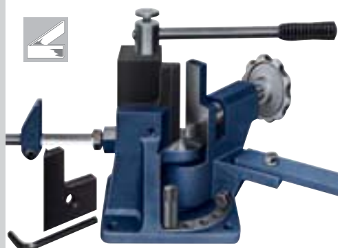
Hoekbuiger WB 100-het origineel! Tot vlakstaal 100 x 6 mm
