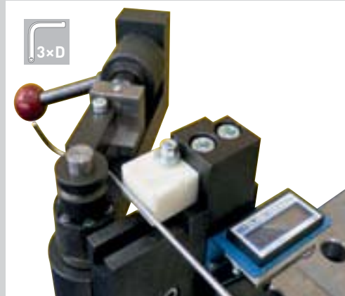
Manuele buizenbuiger HRB 15 tot dia. 15 mm
