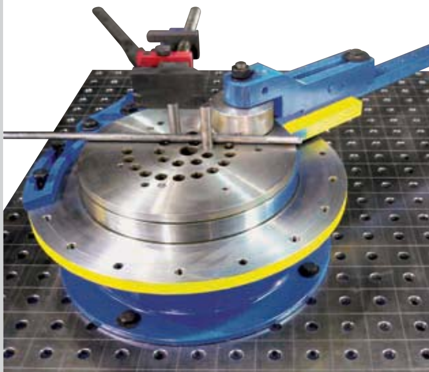
Universele manuele buiger. Om vlakstaal te buigen, staaf of buis tot D = 33 mm
